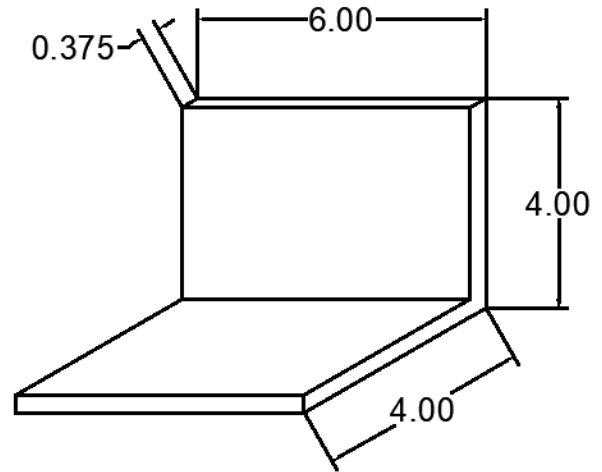
6 ANC-4406-6 ANCHOR CLIP
