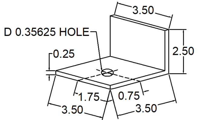
313 ANC-3525-313 DEAD LOAD CLIP
