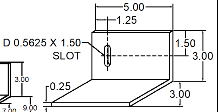
273 STL-3620-273 WIND LOAD CLIP
