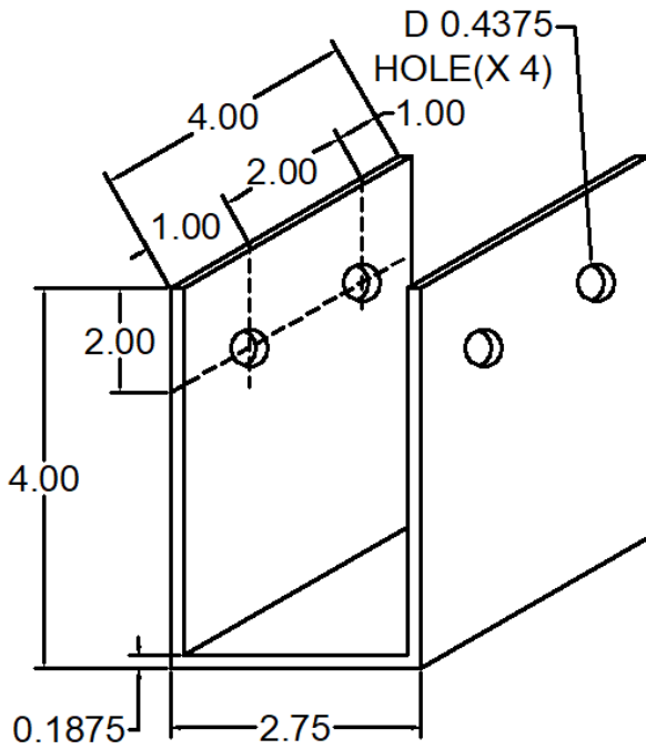
172 ANC-4423-MK-1-172 MULLIAN WRAP
