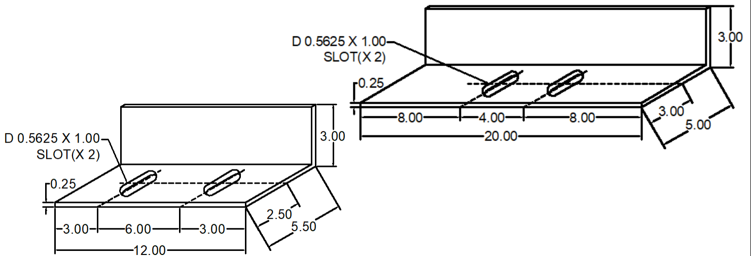
270 STL-3612-270 WIND LOAD CLIP
