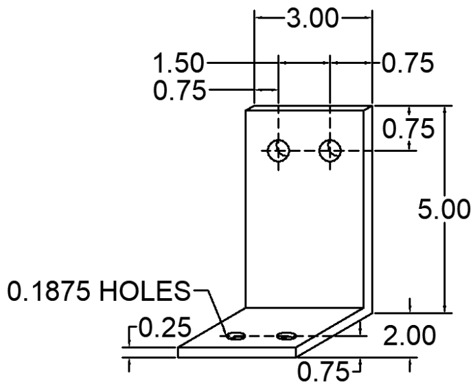
130 ANC-0203-5-130 DEAD LOAD CLIP
