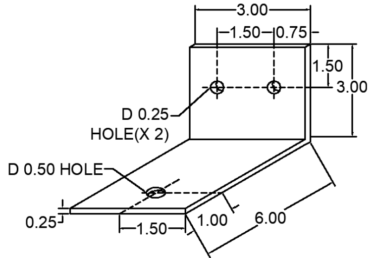
117 ANC-0306-117 DEAD LOAD CLIP
