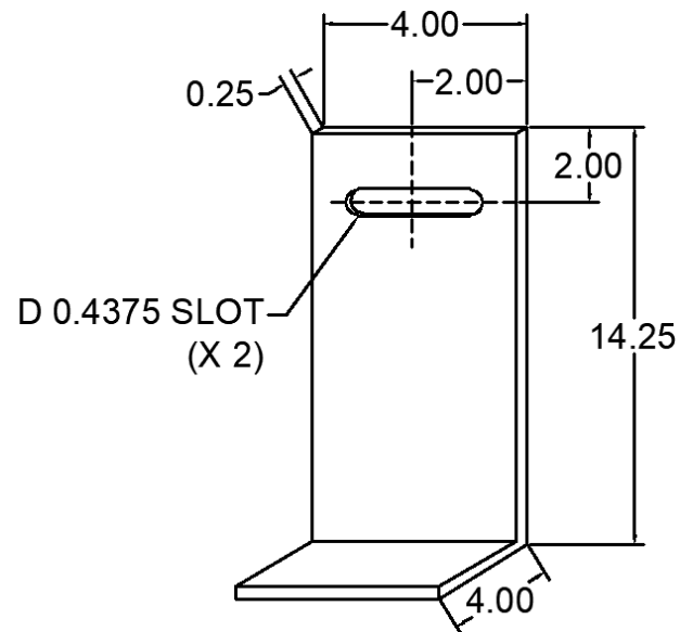
68 ANC-4144-SL-68 WIND LOAD CLIP
