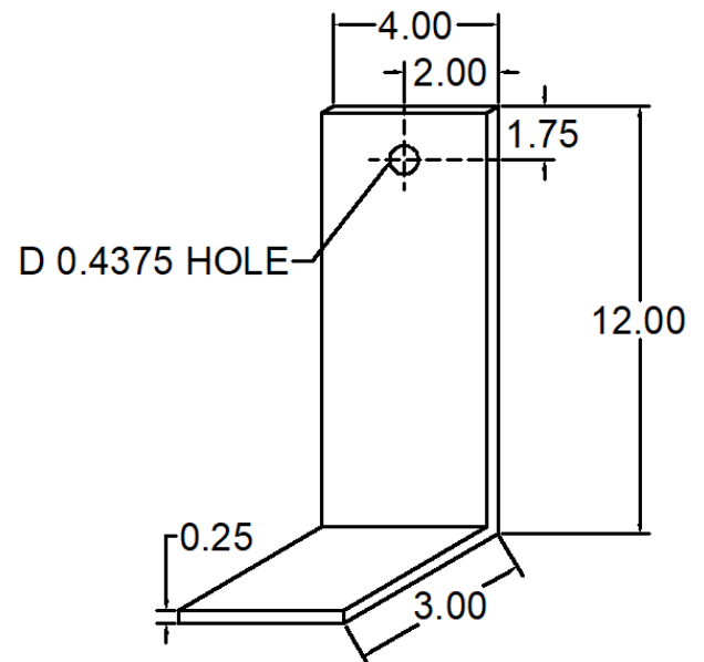
245 ANC-4203-245 WIND LOAD CLIP
