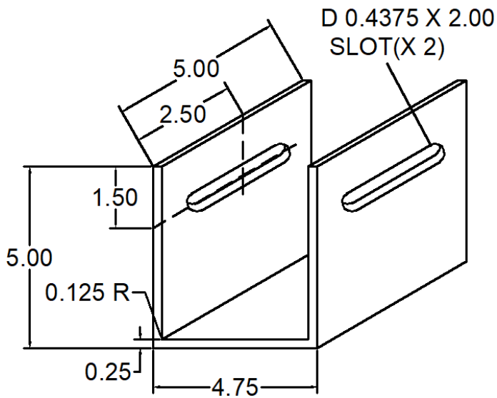
157 ANC-4755-WA-157 MULLIAN WRAP
