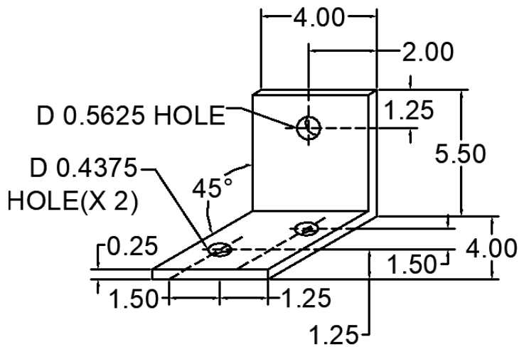
120 ANC-0405-4DL-120 DEAD LOAD CLIP
