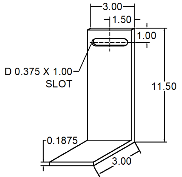
241 ANC-1133-241 WIND LOAD CLIP
