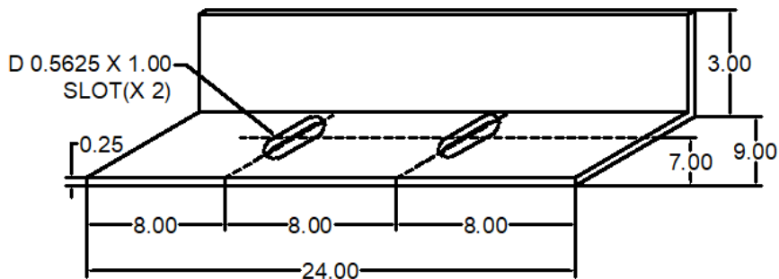
274 STL-3924-274 WIND LOAD CLIP
