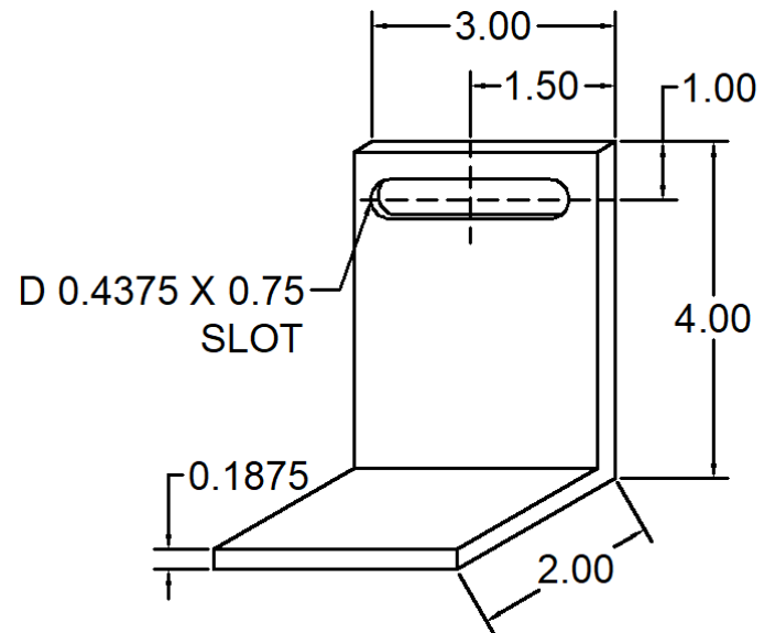
245 ANC-4203-245 WIND LOAD CLIP
