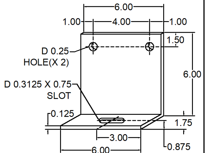
259 ANC-1766-259 WIND LOAD ANCHOR
