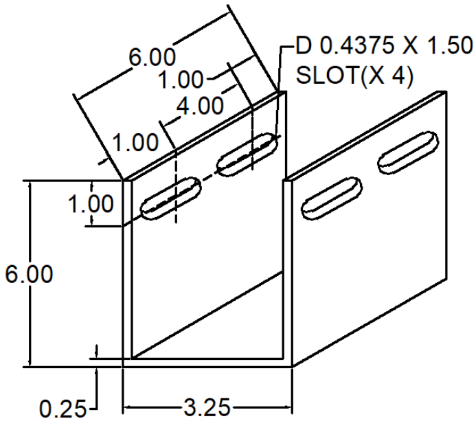
165 ANC-0206-6-165 MULLIAN WRAP
