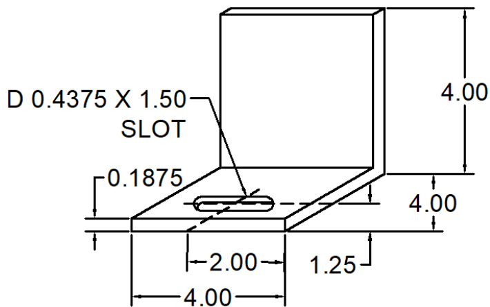
242 ANC-4404-242 WIND LOAD CLIP
