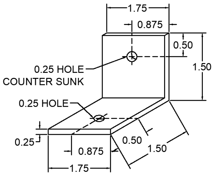
73 ANC-15175-73 DEAD LOAD CLIP
