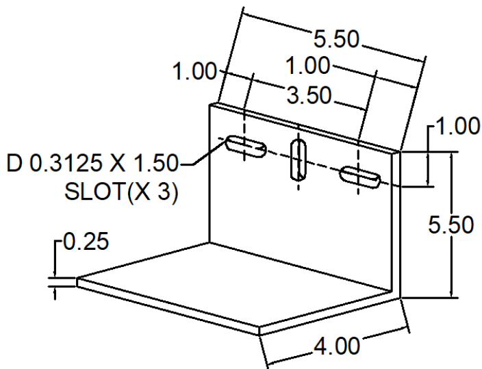
317 WLA-0404-317 WIND LOAD CLIP
