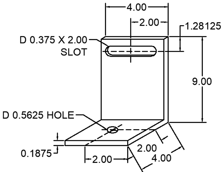
98 ANC-0904-4-98 WIND LOAD CLIP
