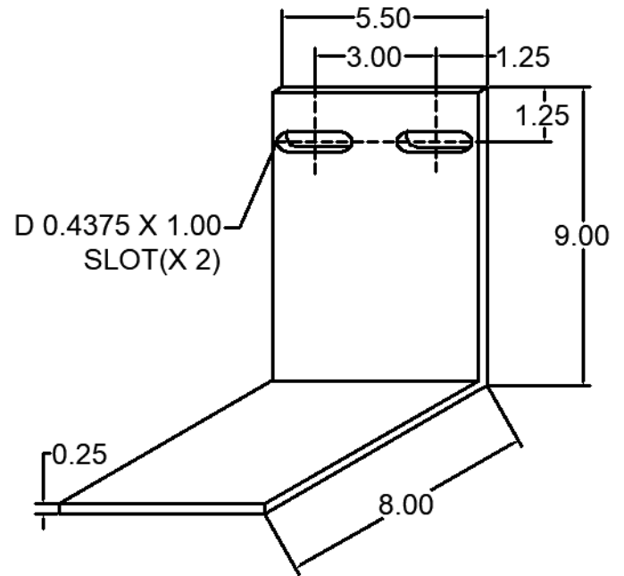
113 ANC-0809-55-113 WIND LOAD CLIP
