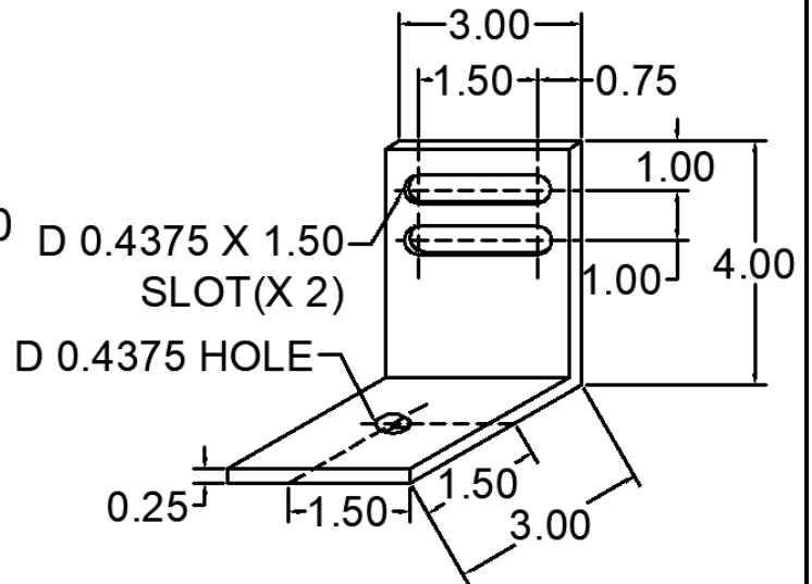
113 ANC-0809-55-113 WIND LOAD CLIP
