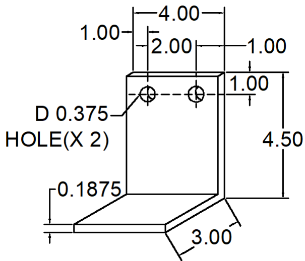
252 ANC-4534-252 DEAD LOAD ANCHOR
