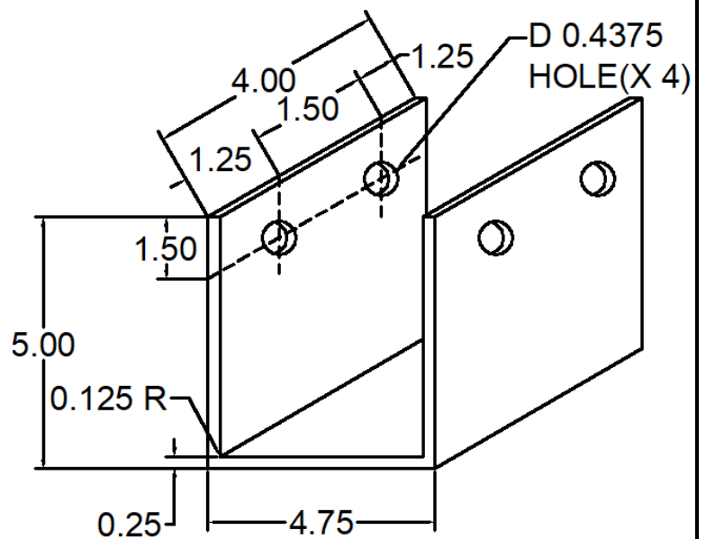
169 ANC-3441-169 MULLIAN WRAP
