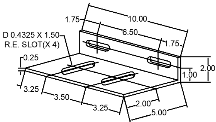
222 ANC-2510-222 WIND LOAD CLIP
