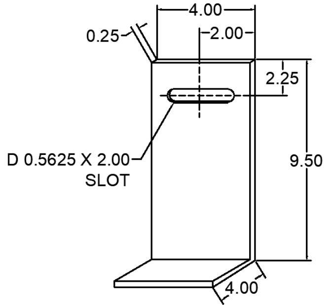
70 ANC-0404-9WCM-70 WIND LOAD CLIP
