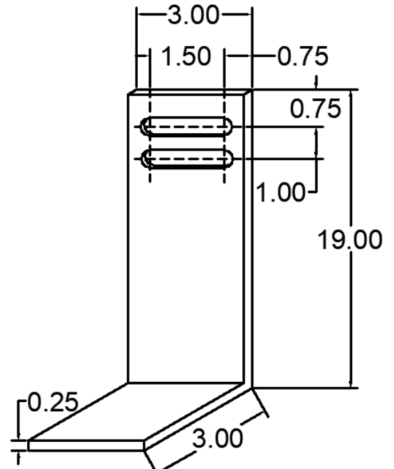
103 ANC-0303-19-103 WIND LOAD CLIP
