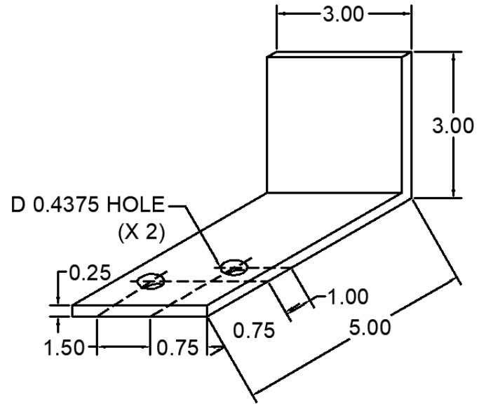
86 ANC-0303-5-86 DEAD LOAD CLIP
