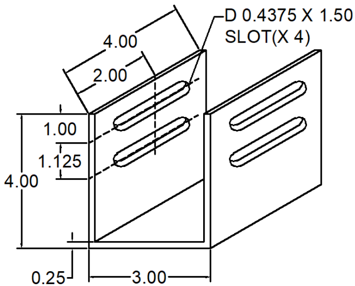
168A ANC-3442-168A MULLIAN WRAP
