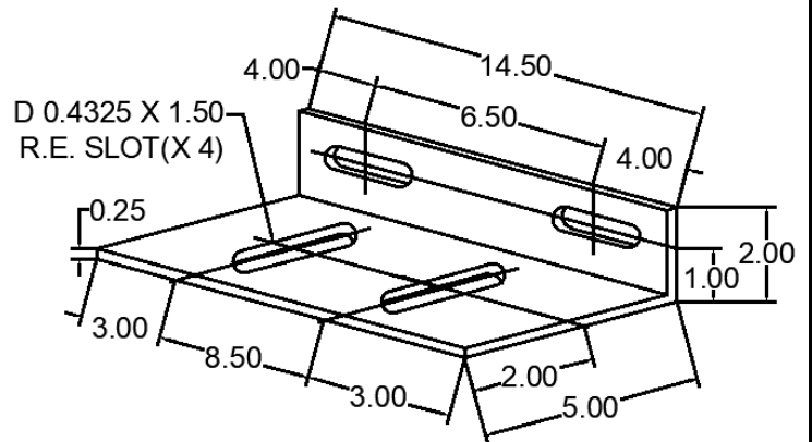
223 ANC-2514-223 WIND LOAD CLIP
