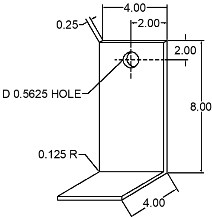
59 ANC-0404-8DL-59 DEAD LOAD CLIP
