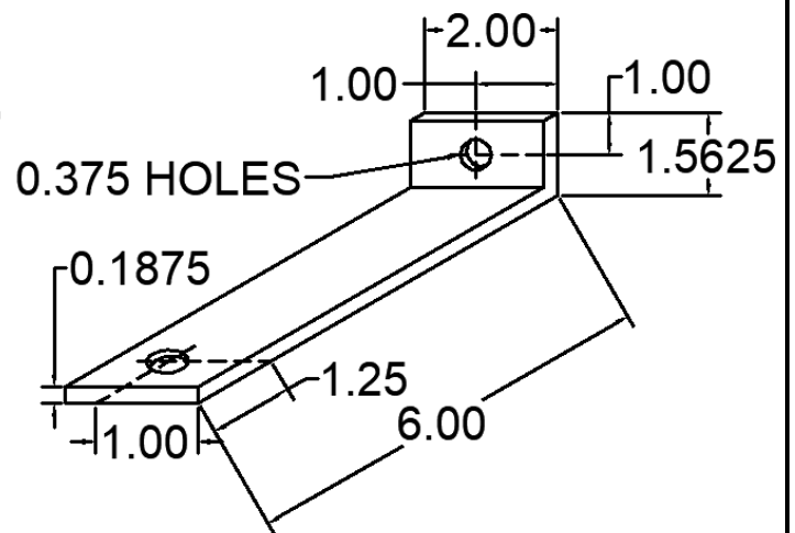
92 ANC-1602-M-92 DEAD LOAD CLIP
