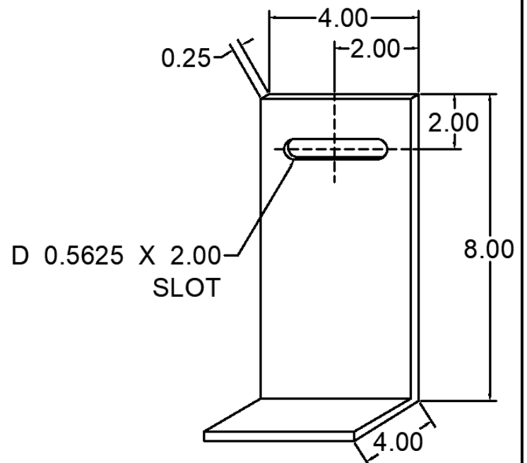
60 ANC-0404-8WL-60 WIND LOAD CLIP
