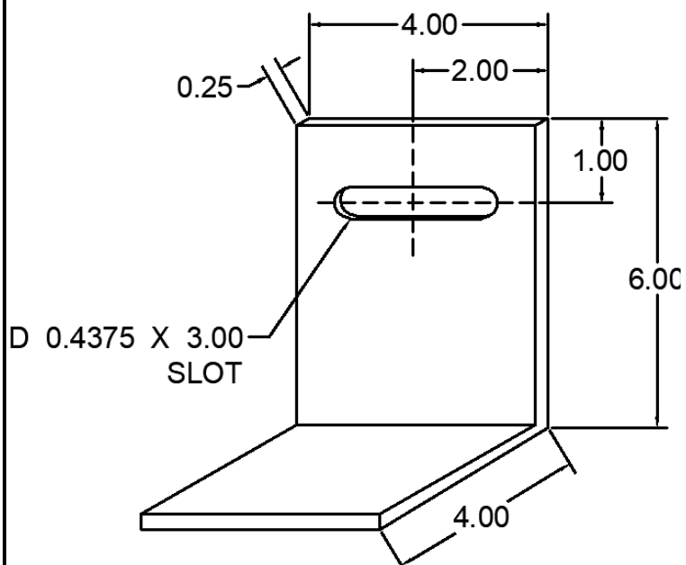
39 ANC-0001-39 WIND LOAD CLIP
