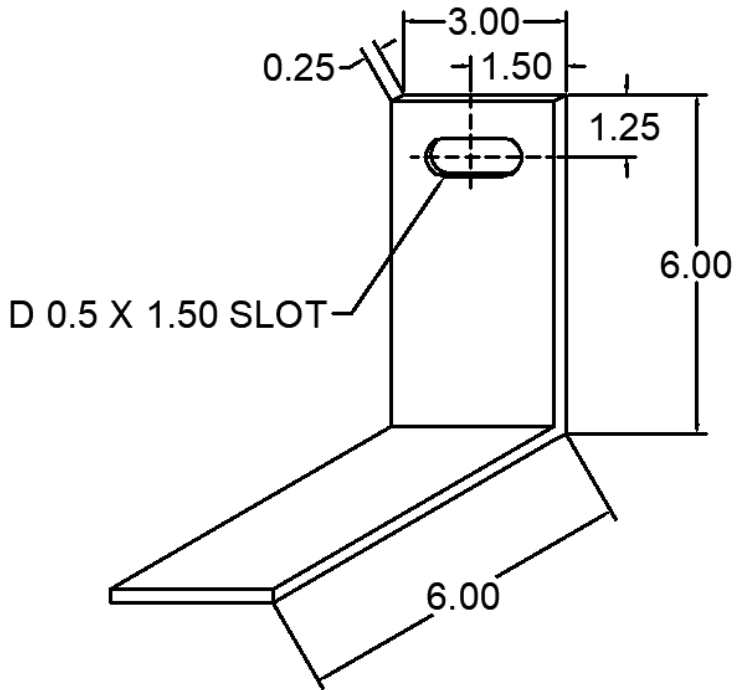
49 ANC-0306-49 WIND LOAD CLIP
