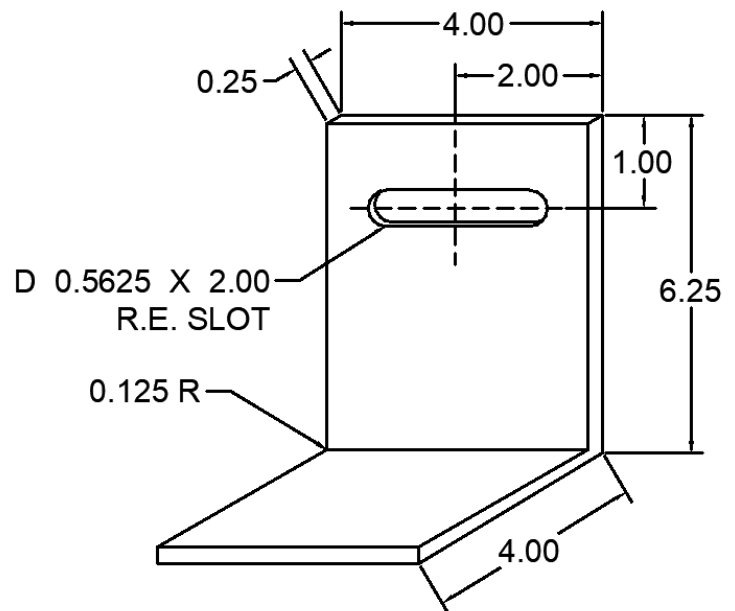
44 ANC-0406-4WL-44 WIND LOAD CLIP
