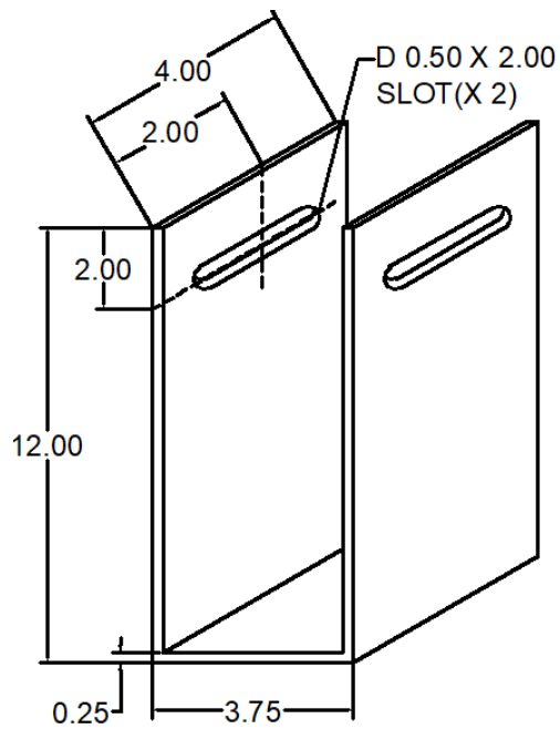
161 ANC-0412-M-161 MULLIAN WRAP
