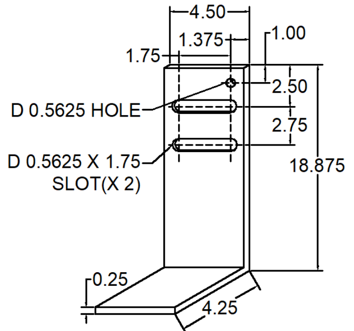
299 ANC-4519-299 WIND LOAD CLIP
