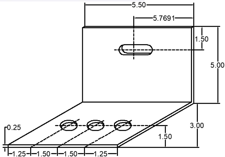
139 ANC-0305-8WL-139 WIND LOAD CLIP
