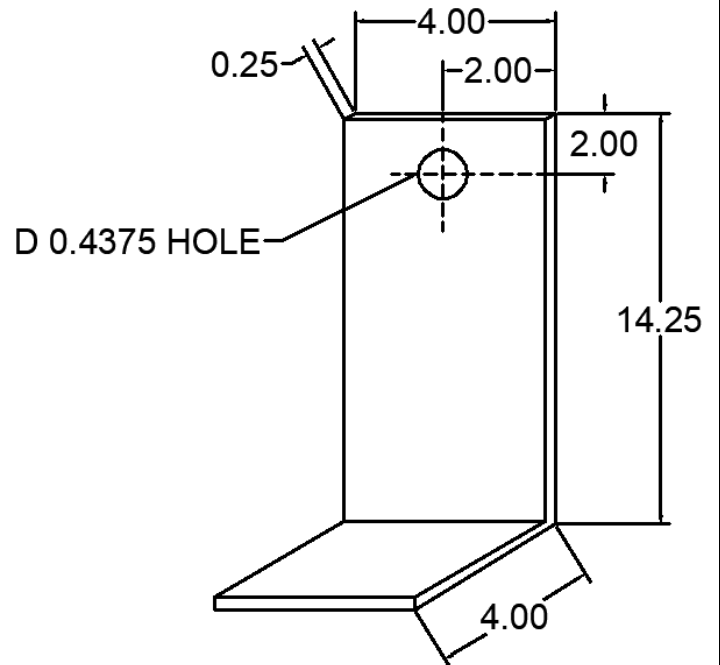
66 ANC-4144-1-10-66 DEAD LOAD CLIP
