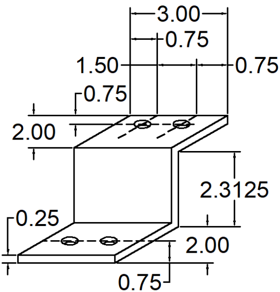
185 ANC-0203-ZM-185 OFFSET DEAD LOAD TOP
