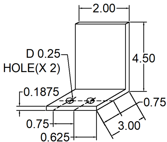
254 ANC-3402-254 DEAD LOAD CLIP
