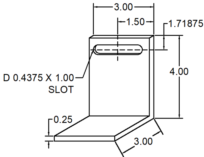
244 ANC-4303-244 WIND LOAD CLIP
