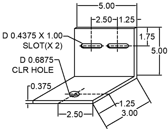
116 ANC-0001-116 WIND LOAD CLIP
