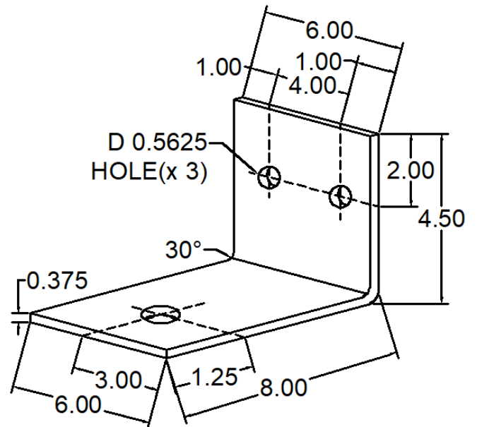
297 ANC-4586-297 DEAD LOAD CLIP
