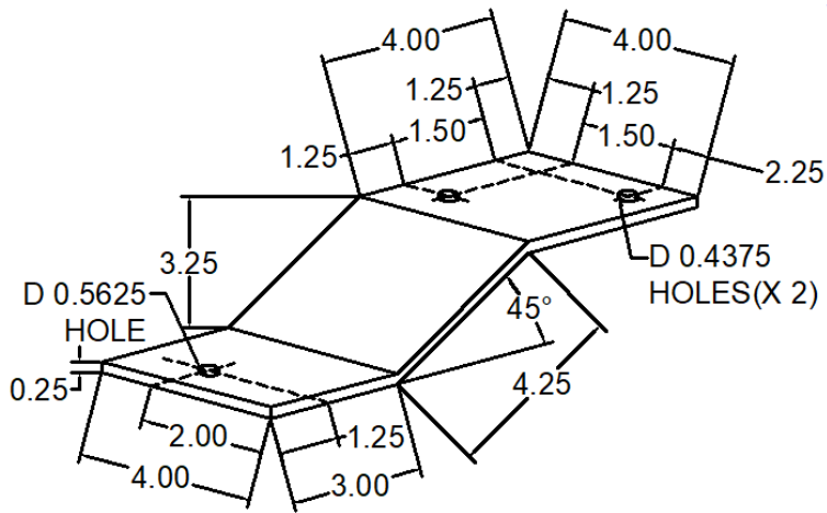
191 ANC-0410-DL-191 DEAD LOAD CLIP
