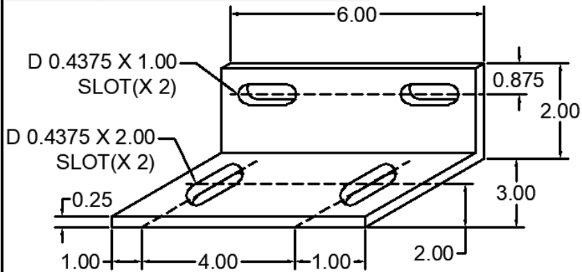
136 ANC-6250-136 WIND LOAD CLIP
