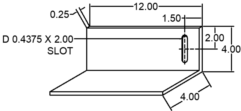
61 ANC-4412-61 WIND LOAD CLIP
