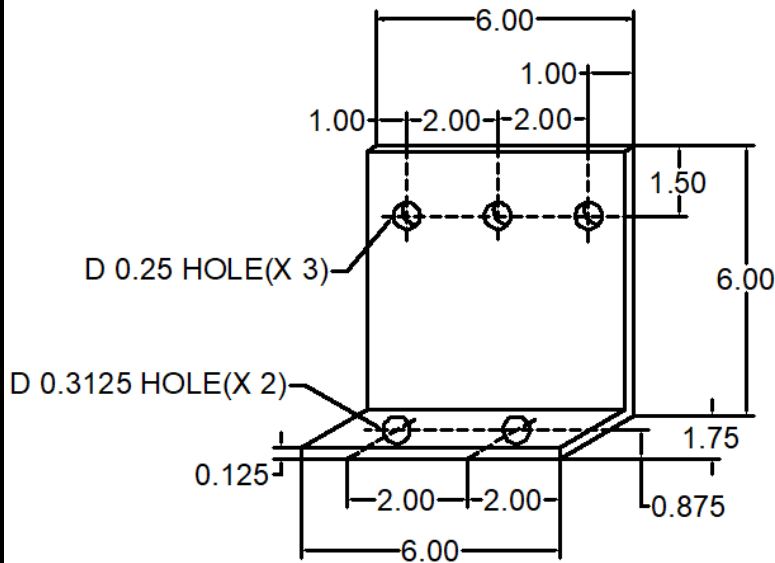
262 ANC-1766-262 DEAD LOAD ANCHOR
