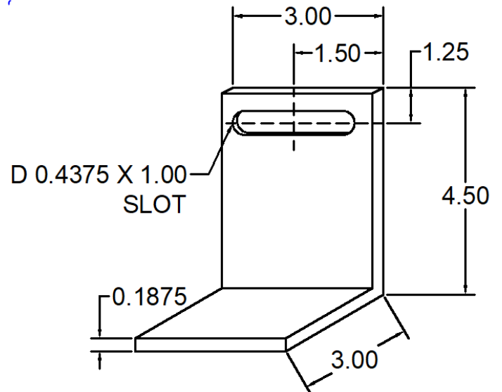
243 ANC-4533-243 WIND LOAD CLIP
