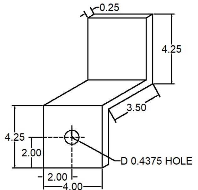
180 ANC-0404-WLZ-180 DEAD LOAD HANGER
