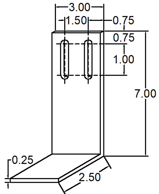
99 ANC-0703-99 WIND LOAD CLIP
