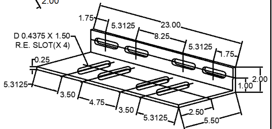
224 ANC-2523-224 WIND LOAD CLIP
