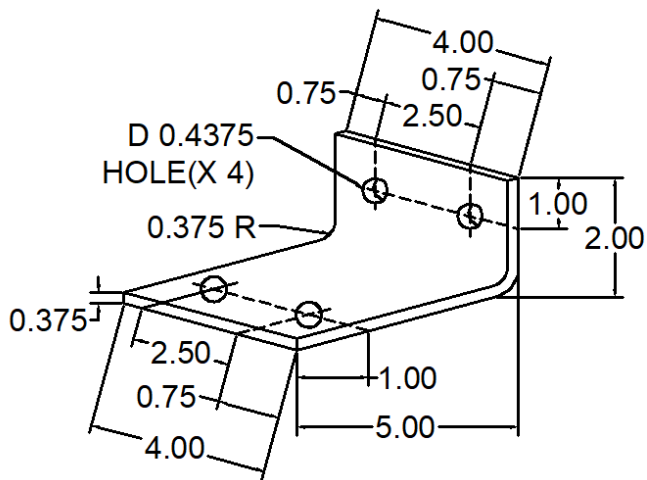
264 ANC-5204-264 DEAD LOAD ANCHOR
