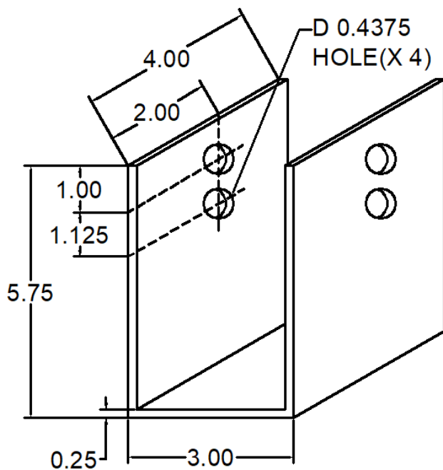
168A ANC-3442-168A MULLIAN WRAP
